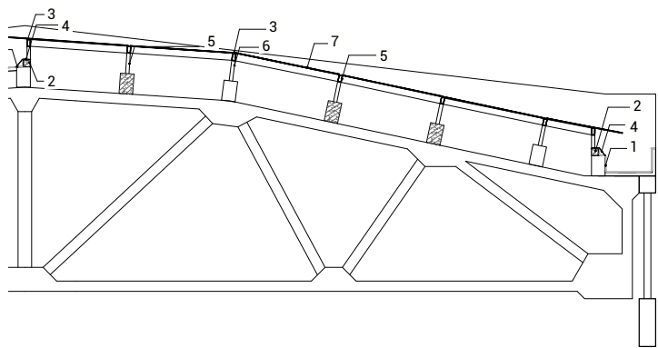
天窗细部
