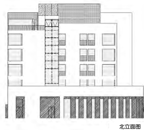
北立面图
