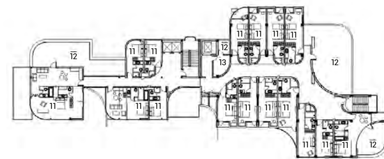
六层平面图
