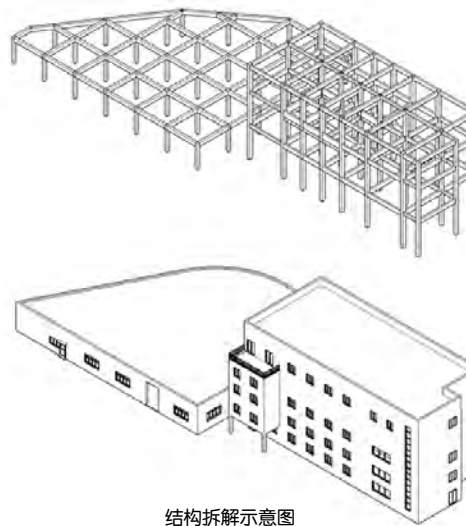
结构拆解示意图
