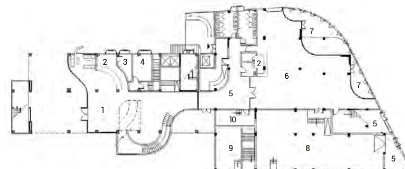
一层平面图
